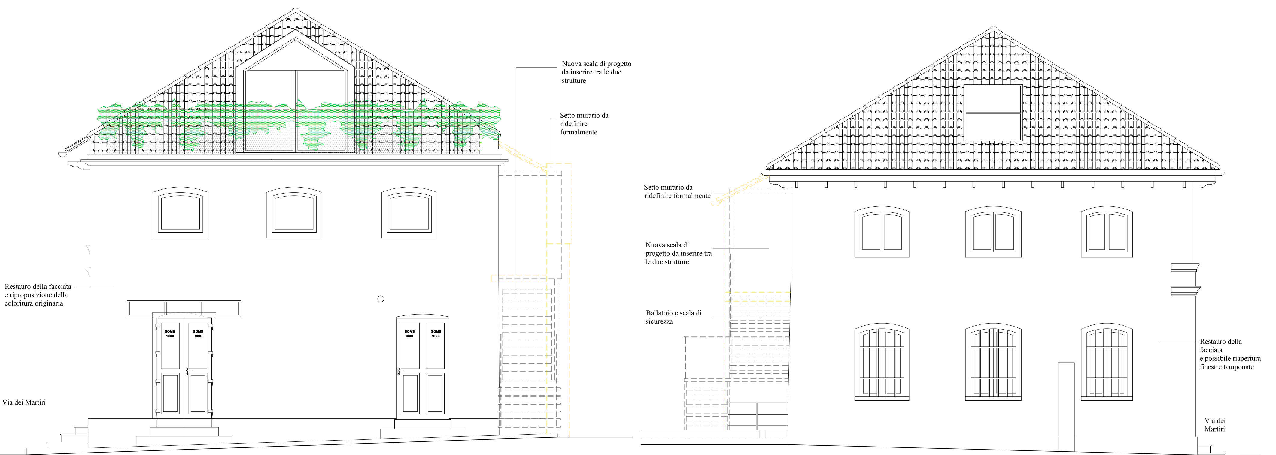
Prospetto ovest - scala 1:50
